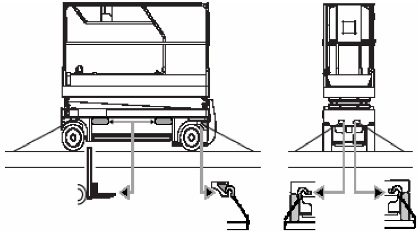
Рисунок 15. Схема строповки и постановки вилочного подхвата.
